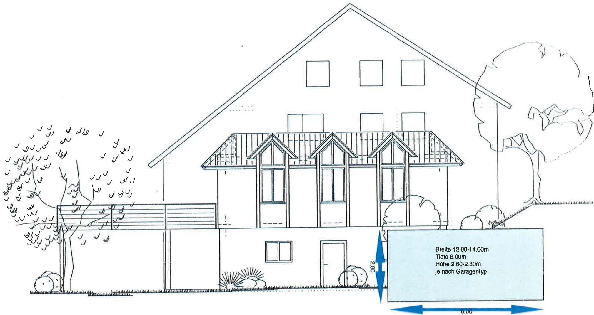
OST-ANSICHT
